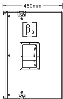
侧视图
