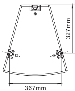
俯视图
